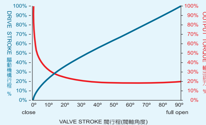
曲柄式驅動機構-行程&扭力曲線圖
