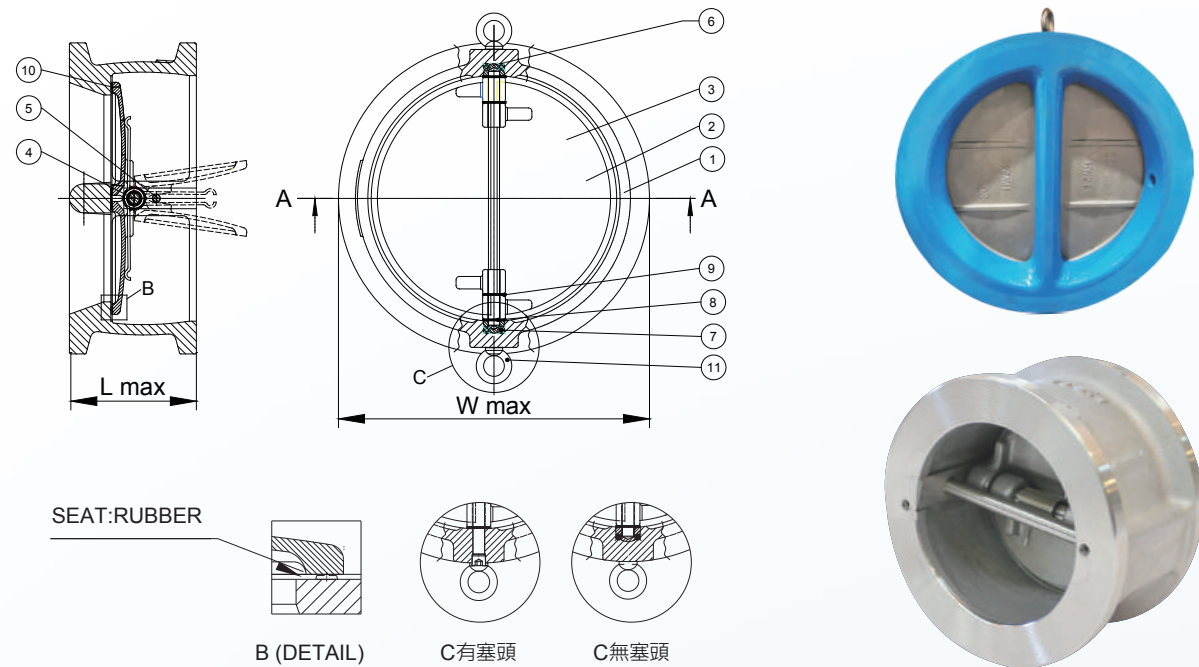
DIMENSION 尺寸表
