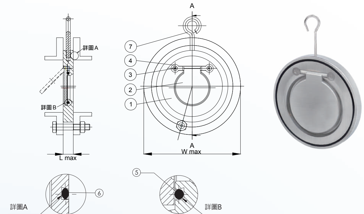
DIMENSION 尺寸表
