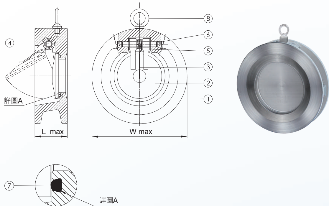
DIMENSION 尺寸表
