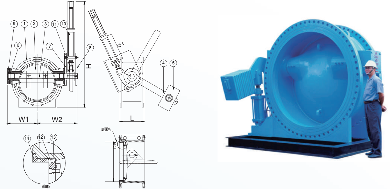
DIMENSION 尺寸表
