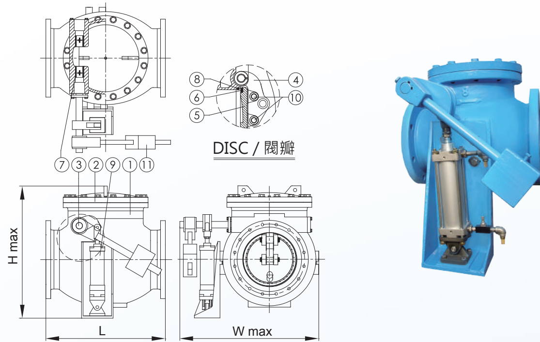
DIMENSION 尺寸表
