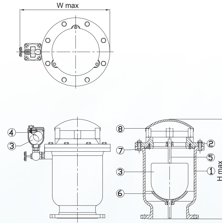
DN200-400 DIMENSION 尺寸表
