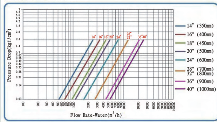
PISTON TYPE / 汽缸型
